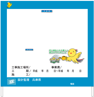
兵庫県養父土木・新温泉土木仕様 木枠看板 ●サイズ:H1800mm以上× W1700mm以上(脚300mm) ●材質:木枠トタン・間伐材製(脚付)
