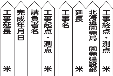
竣工杭(開発局タイプ1) 8072101 ●サイズ:H1800×W90×D90mm
