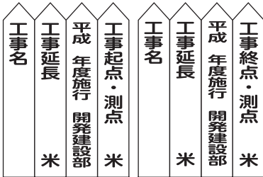
竣工杭(開発局タイプ2) 8072102 ●サイズ:H1800×W90×D90mm
