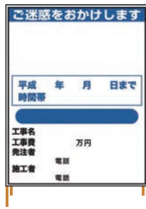
広島県仕様工事看板 ●サイズ:H1400×W1100mm 無反射/プリズム高輝度反射
