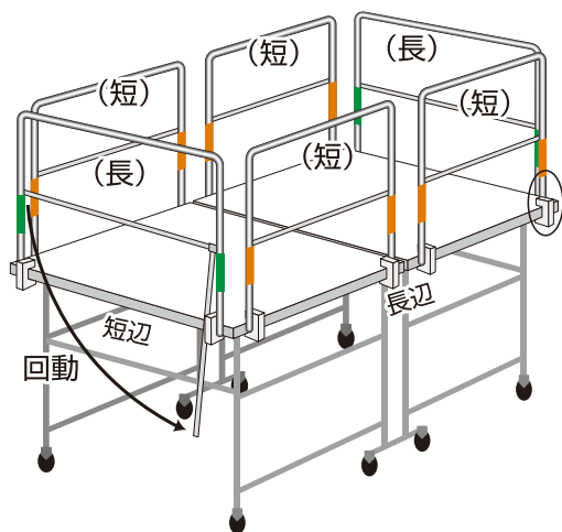
LLタイプ単体使用時手すり取付図
