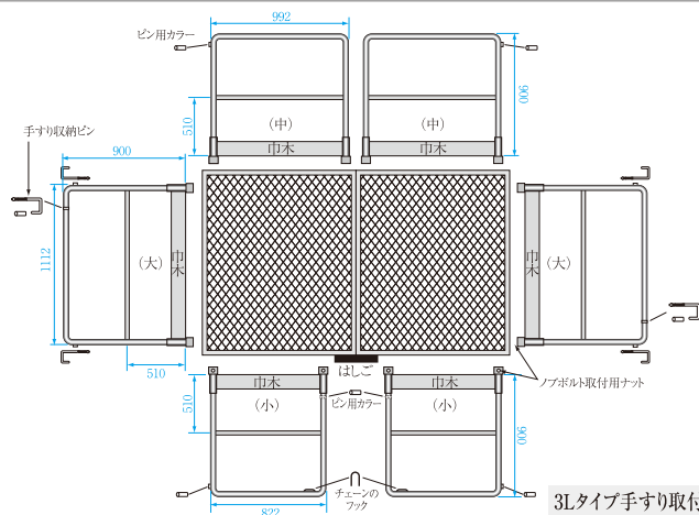
3Lタイプ手すり取付図
