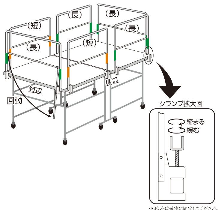
Lタイプ単体使用時手すり取付図
