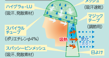
構造図・気化熱の仕組み
