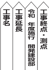
8072102 竣工杭（開発局タイプ2） サイズ H1800×W90×D90mm
