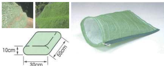
6492010 植生土のう
